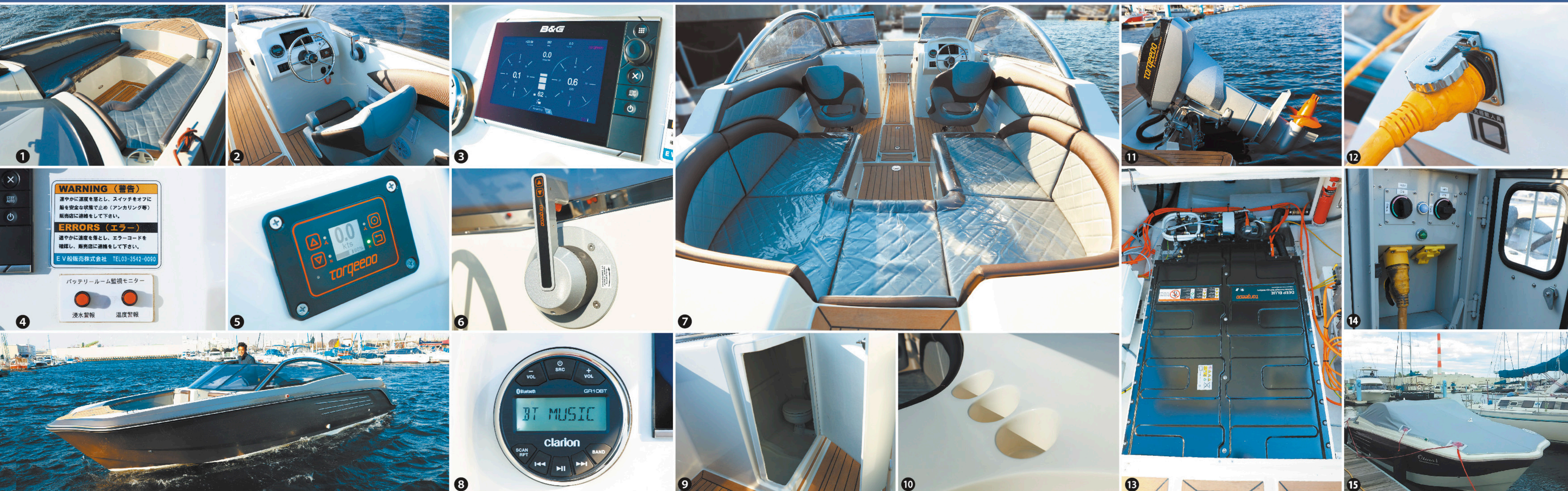
①バウ側シート ②運転席 ③モニター&コントロールパネル ④バッテリールーム監視モニター ⑤トルキードサブモニター ⑥コントロールレバー ⑦リアシート ⑧マリンオーディオ ⑨トイレ ⑩ドリンクホルダー ⑪トルキードエレクトリック船外機 ⑫船体側充電ポート ⑬高電圧バッテリー ⑭充電設備(参考) ⑮船体カバー(オプション) ※オプション: ボディカラー、ウッドデッキ、船底塗装
